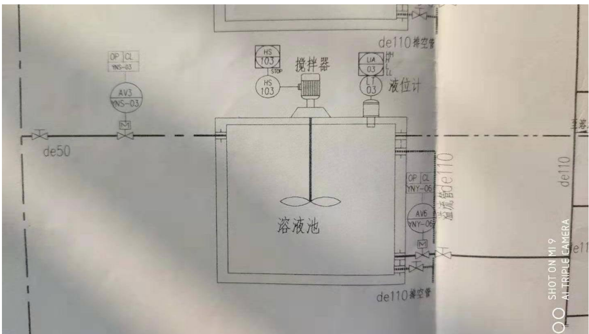
(下图为溶液池纵剖面图)
